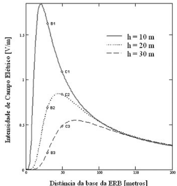
Figura 5 - Intensidade de campo elétrico em função da distância x da base da ERB considerando três diferentes alturas de instalação da antena.
